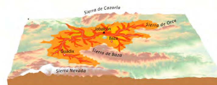
Reconstrucción paleogeográfica de la evolución de la cuenca de Guadix-Baza.
