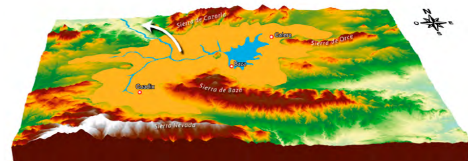
CAPTURA DE LA CUENCA POR EL RÍO GUADALQUIVIR
